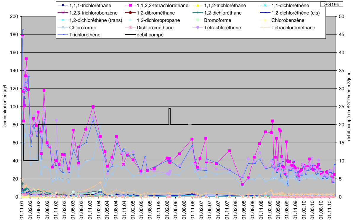
Figure 2 : Suivi du pompage en SG19b, évolution des concentrations dans l'eau pompée. Données depuis 2001.
