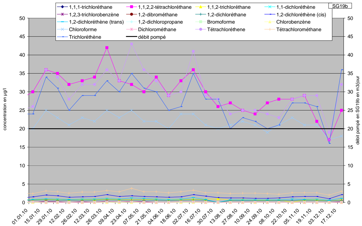
Figure 3 : Suivi du pompage en SG19b, évolution des concentrations dans l'eau pompée. Données 2010.
