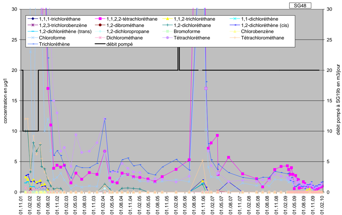
Figure 5 : Suivi du pompage en SG19b, évolution des concentrations en SG48
