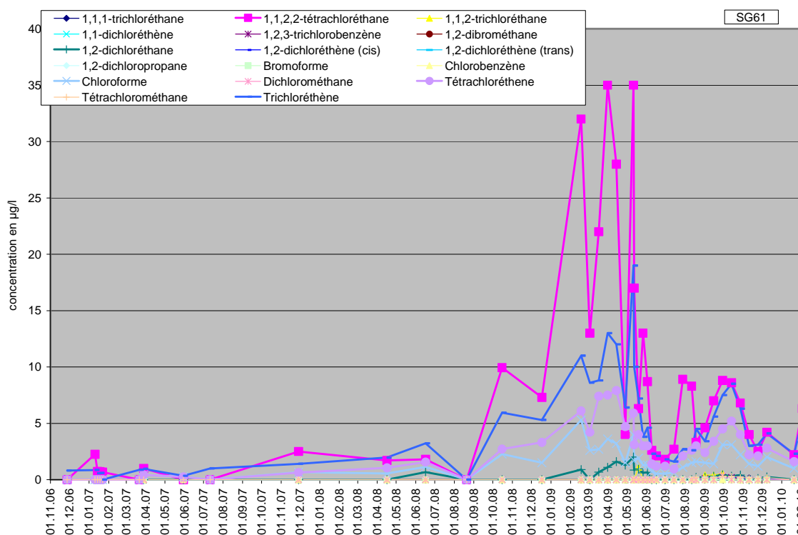
Figure 2 : Suivi du pompage en SG19b, évolution des concentrations en SG61
