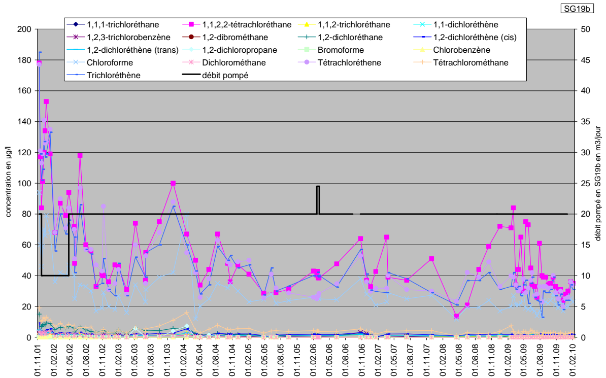
Figure 3 : Suivi du pompage en SG19b, évolution des concentrations dans l'eau pompée
