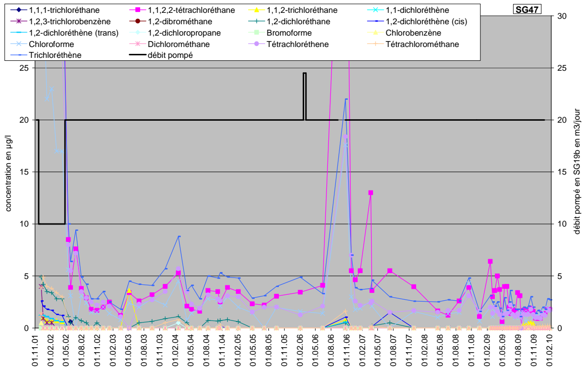
Figure 4 : Suivi du pompage en SG19b, évolution des concentrations en SG47
